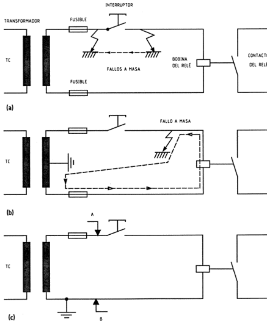
Figura H3 - Protección contra fallos a masa
